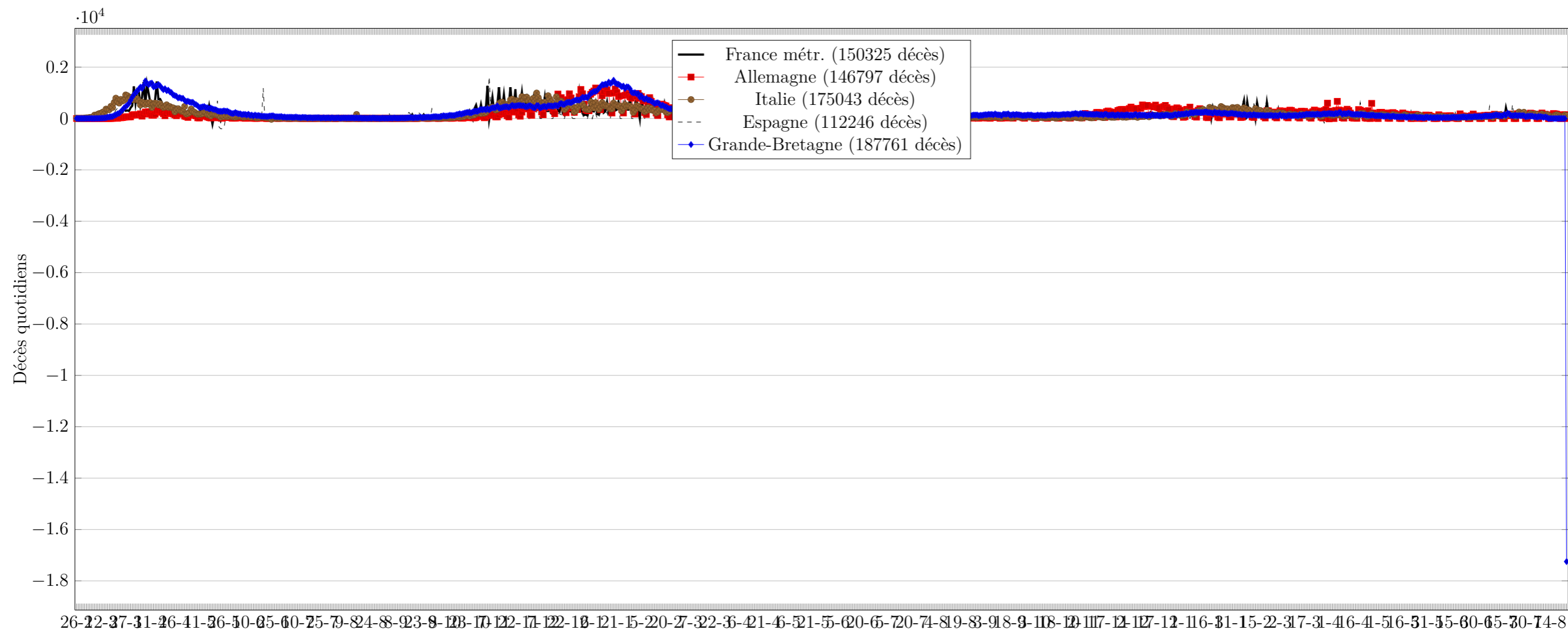
Figure 1 – Nombre de nouveaux décès comptabilisés chaque jour. Les sauts peuvent être liés à de nouvelles modalités de recensement (ex. : intégration des décès en Ehpad le 2 avril pour la France, de leur équivalent en Grande-Bretagne le 29 avril). Ce graphique n'est pas très lisible, mais donne d'emblée l'évolution journalière du phénomène et permet une première comparaison entre pays : Espagne dépassant l'Italie dès le 25 mars, décroissance de ces deux pays (11 avril), statistiques erratiques de la France et en Grande-Bretagne. Mais ces graphiques ne tiennent pas compte de la population des pays. Attention, la valeur de l'Allemagne le 11 avril est bizarre (négative, cf. ma remarque dans l'introduction). De même pour celle de la France le 16 mai (2 morts négatifs ; Le Monde annonce néanmoins 27625 décès au total, quand Hopkins en affiche 27483). Il ne faut donc pas s'inquiéter outre mesure du brutal excès de décès le 17 mars, qui compense l'oubli de la veille. Ni des 200 morts négatifs du 19 mai. De même pour les 1800 résurrections espagnoles du 25 mai, étalées par mes soins sur 3 jours pour ne pas changer brutalement l'allure des courbes. Ici, la généalogie critique des chiffres et des organisations qui les publient est d'une importance capitale .
