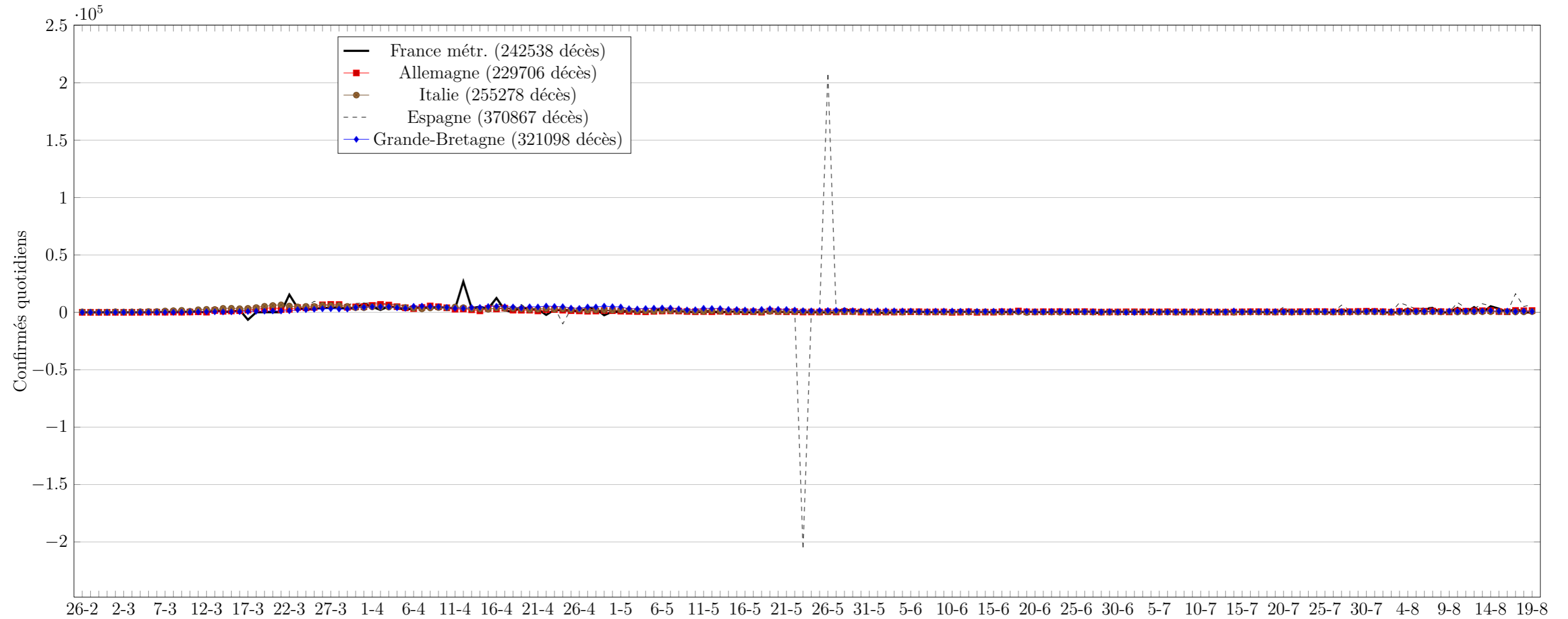
Figure 1 – Nombre de nouveaux confirmés comptabilisés chaque jour. Les sauts peuvent être liés à de nouvelles modalités de recensement (ex. : intégration des décès en Ehpad le 2 avril pour la France, de leur équivalent en Grande-Bretagne le 29 avril). Ce graphique n'est pas très lisible, mais donne d'emblée l'évolution journalière du phénomène et permet une première comparaison entre pays : Espagne dépassant l'Italie dès le 25 mars, décroissance de ces deux pays (11 avril), statistiques erratiques de la France et en Grande-Bretagne. Mais ces graphiques ne tiennent pas compte de la population des pays. Attention, la valeur de l'Allemagne le 11 avril est bizarre (négative, cf. ma remarque dans l'introduction). De même pour celle de la France le 16 mai (2 morts négatifs ; Le Monde annonce néanmoins 27625 décès au total, quand Hopkins en affiche 27483). Il ne faut donc pas s'inquiéter outre mesure du brutal excès de décès le 17 mars, qui compense l'oubli de la veille. Ni des 200 morts négatifs du 19 mai. De même pour les 1800 résurrections espagnoles du 25 mai, étalées par mes soins sur 3 jours pour ne pas changer brutalement l'allure des courbes. Ici, la généalogie critique des chiffres et des organisations qui les publient est d'une importance capitale .
